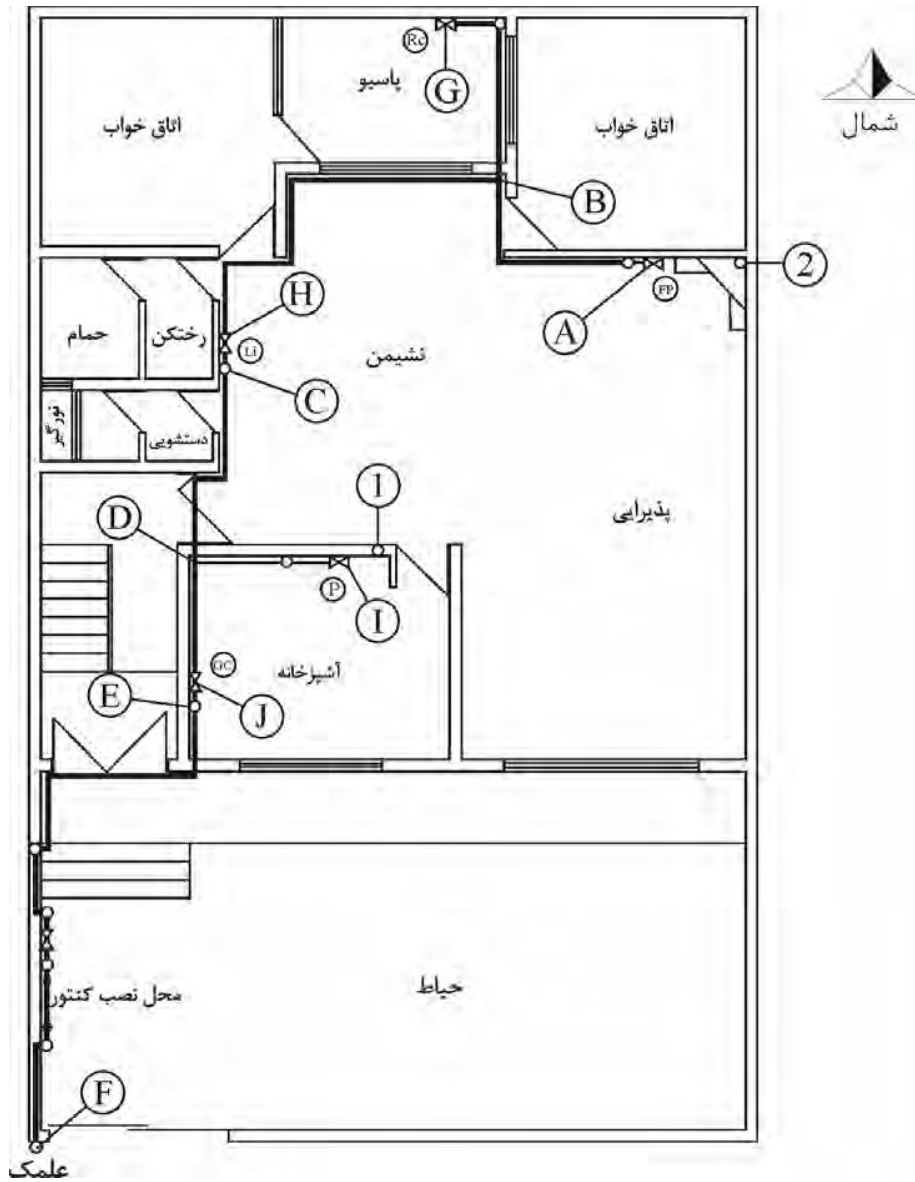
شکل پ-۲-۱ نقشه پلان لوله‌کشی گاز نمونه.
