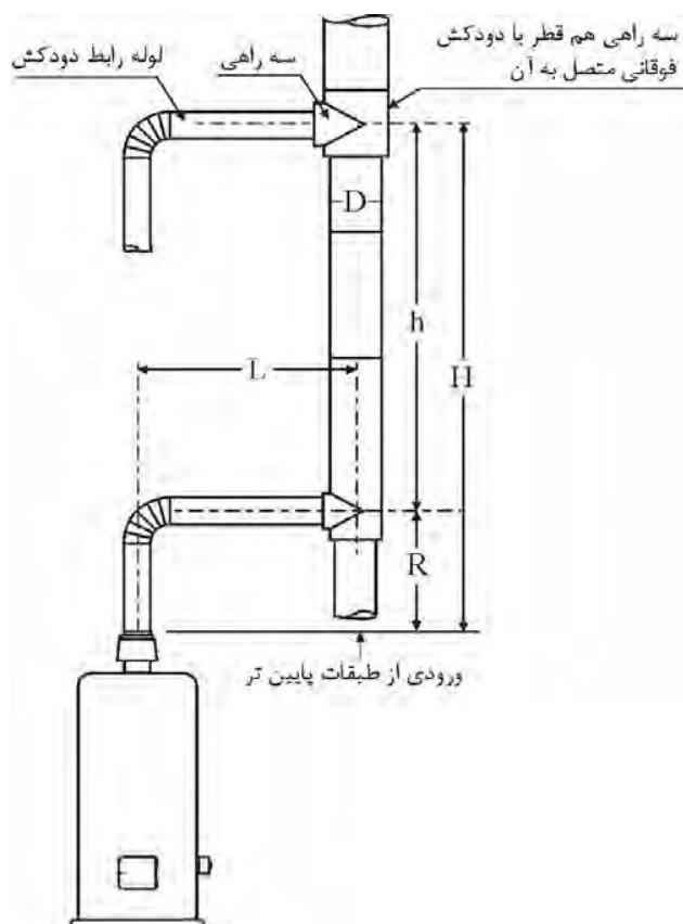
شکل ۳-۸-۱۷ شمای دودکش مشترک ساختمان‌های چندطبقه برای هر قسمت.
